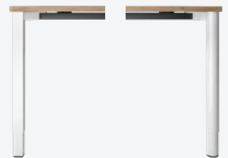
Gestelltyp 4-Fuß Rohr in Rohr Rechts: Rundrohr Links: Quadratrohr Höhenverstellung: 650–880 mm
