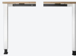
Gestelltyp 4-Fuß Verstellhülse Rechts: Rundrohr Links: Quadratrohr Höhenverstellung: 680–820 mm
